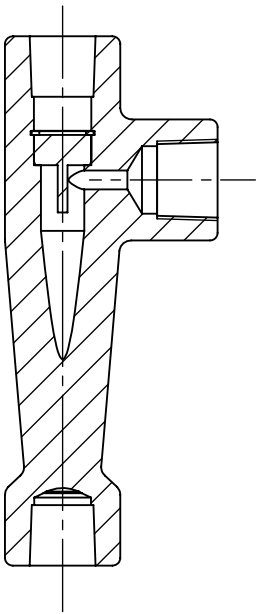
剖面 B-B
