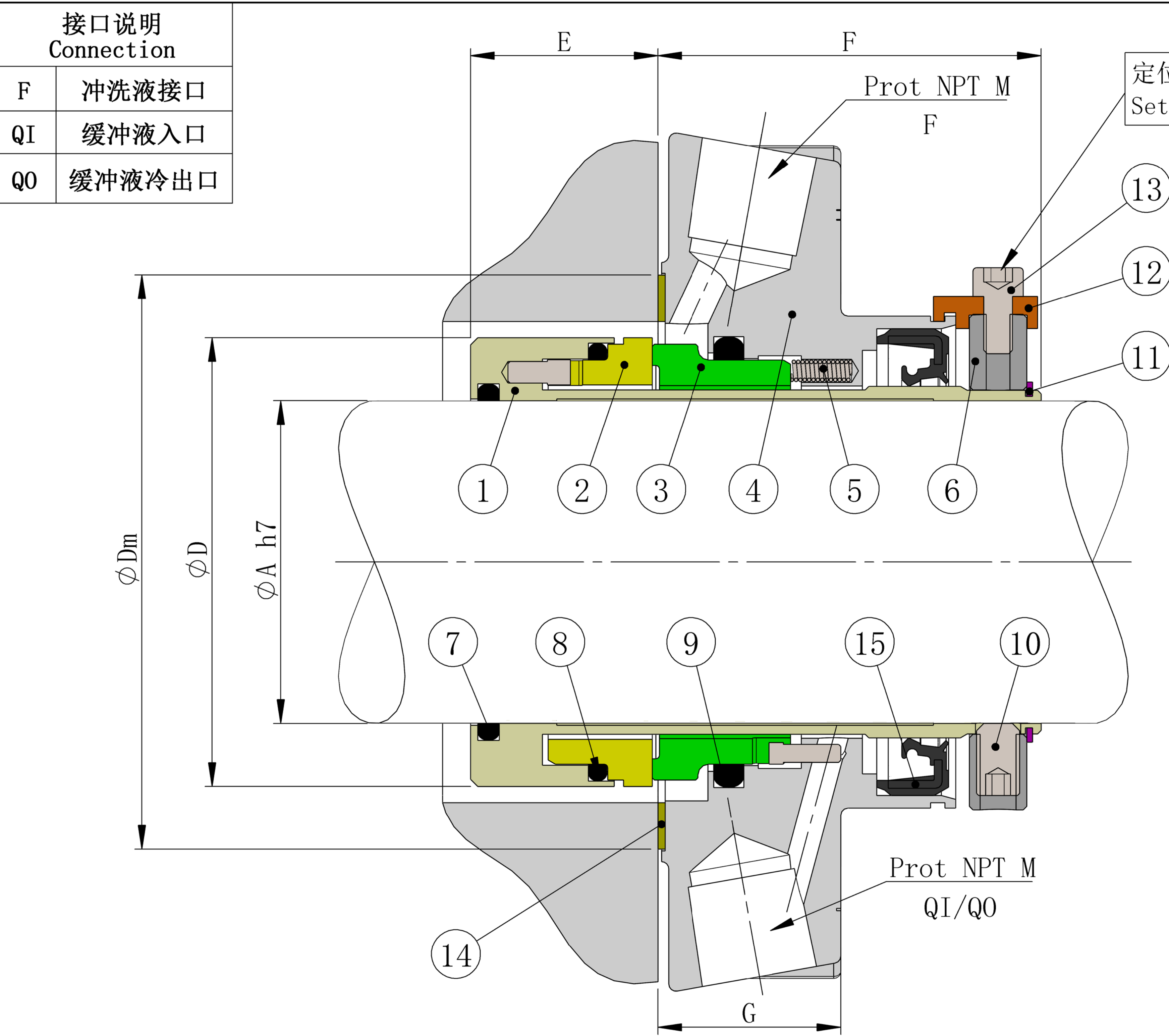
KSCN-尺寸信息（mm）
