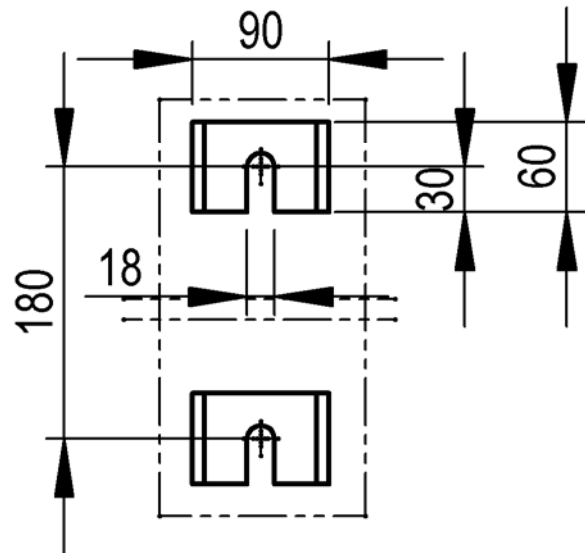
安装尺寸 installation dimension
