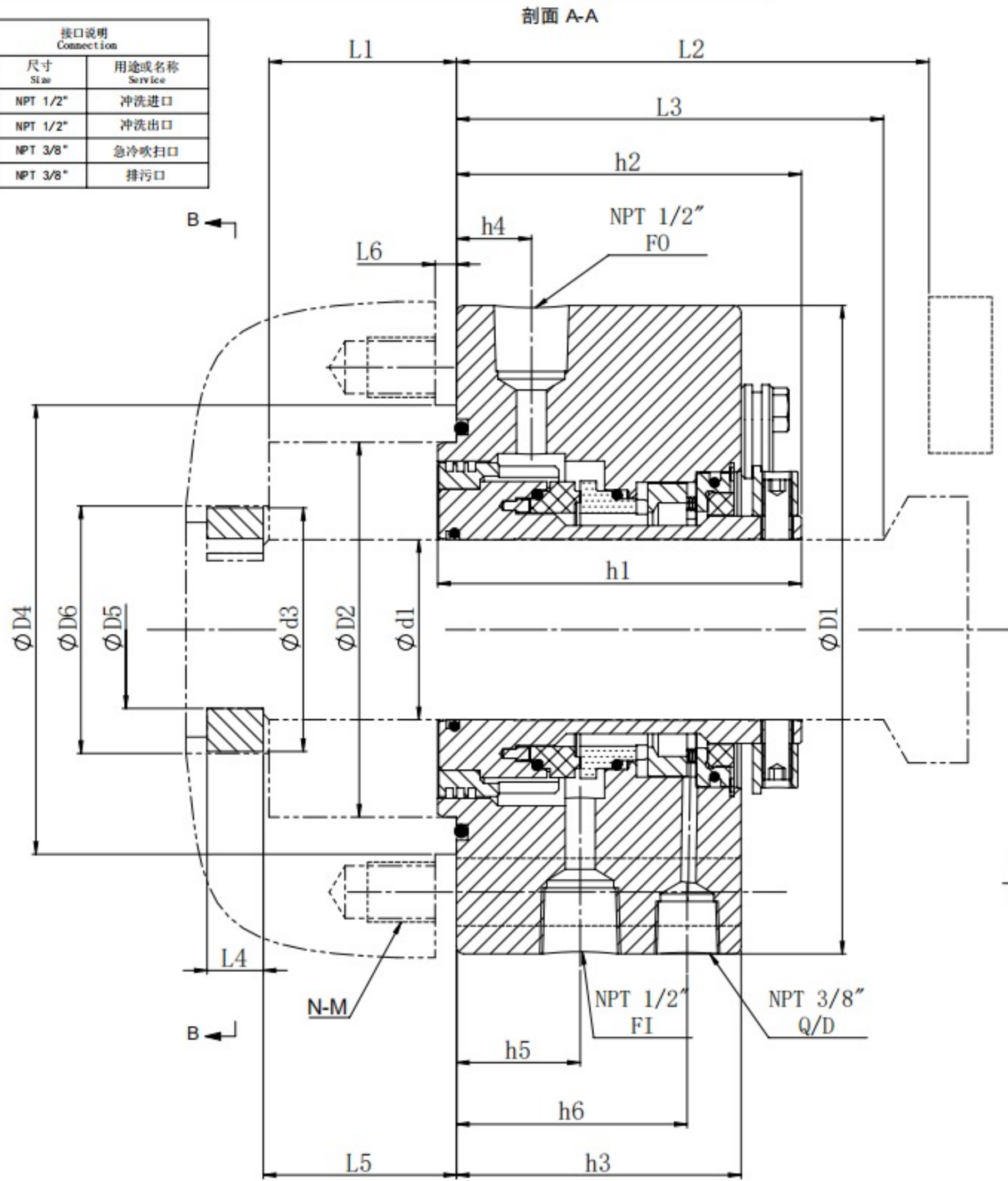
机封尺寸 (FBU填写)
