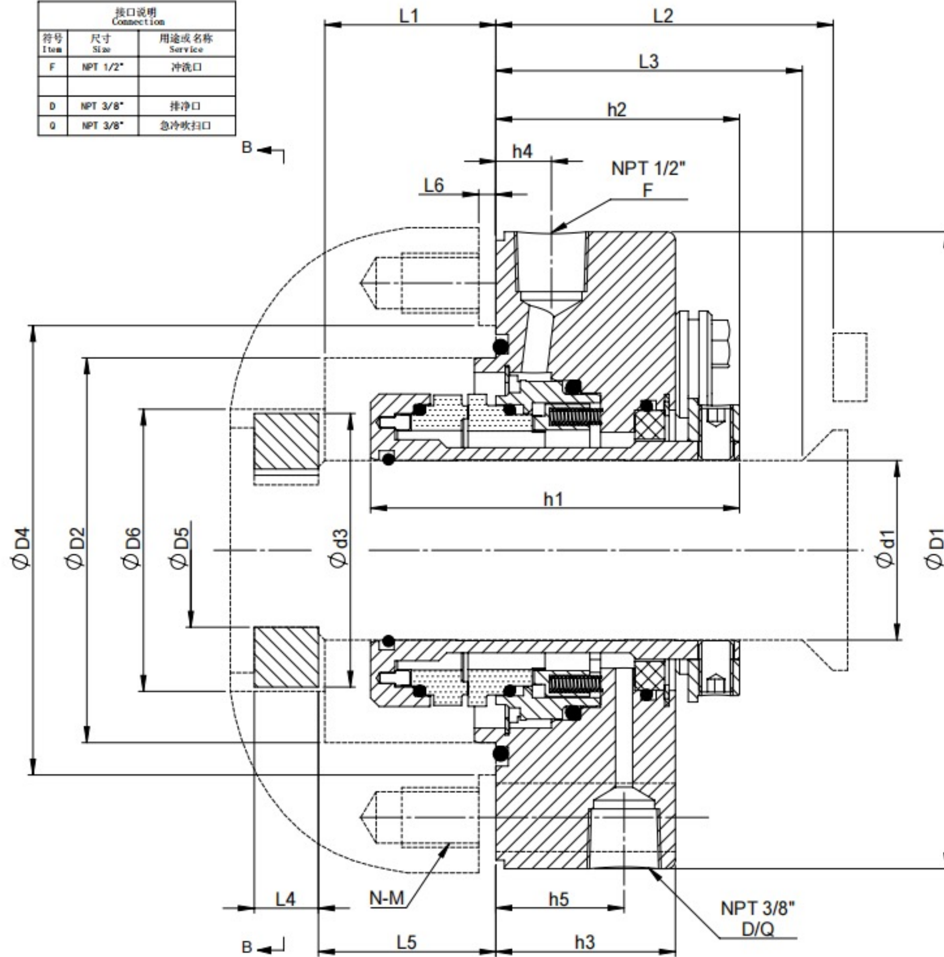
剖面 A-A
