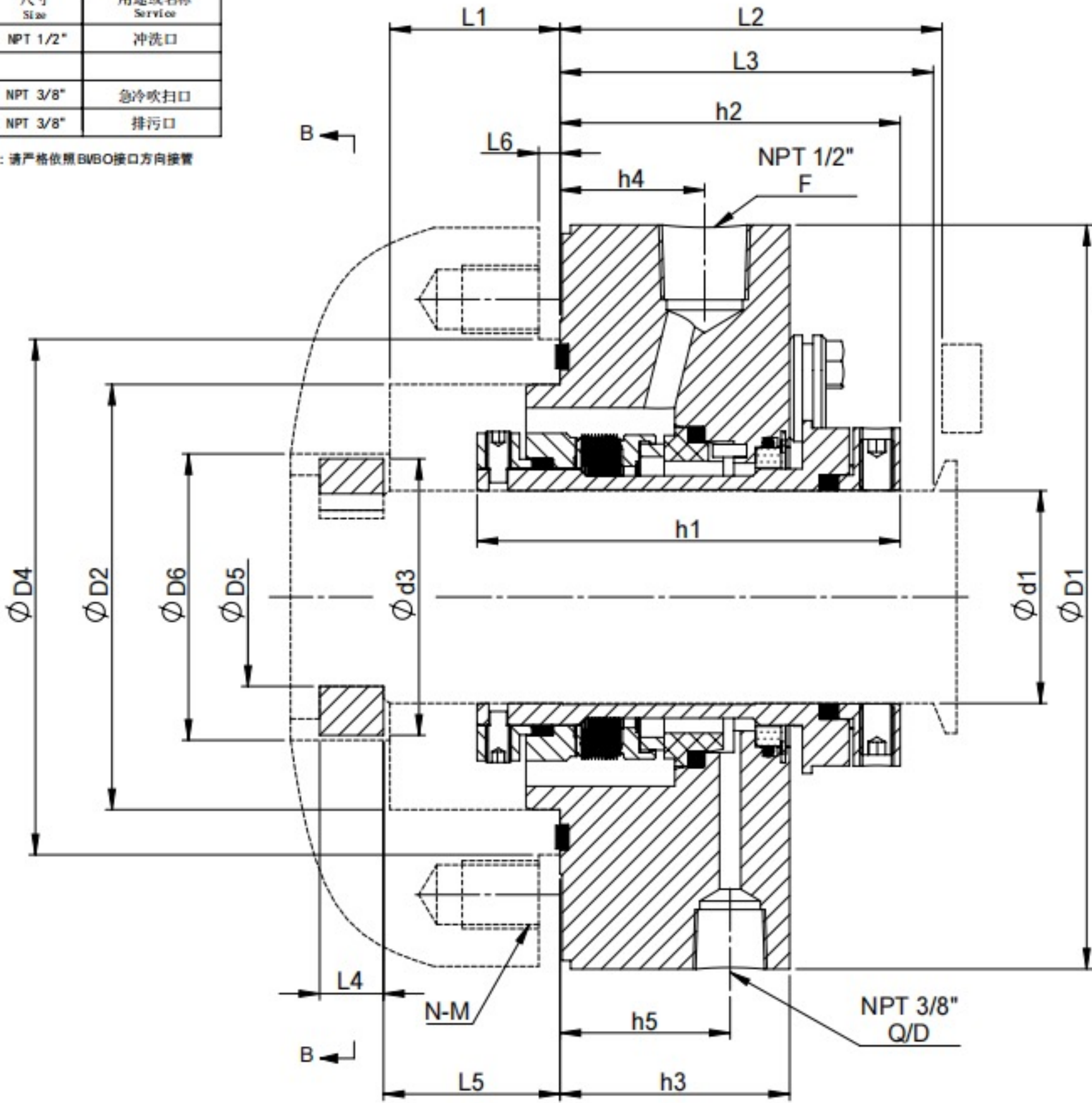
剖面 A-A
