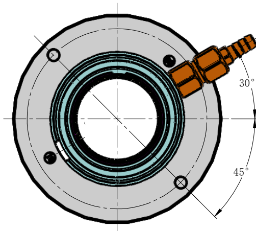
K向/View K 比例不符/NO SCALE
