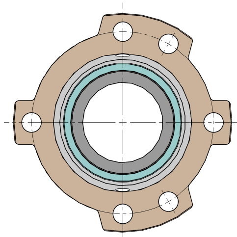
K向/View K 比例不符/NO SCALE
